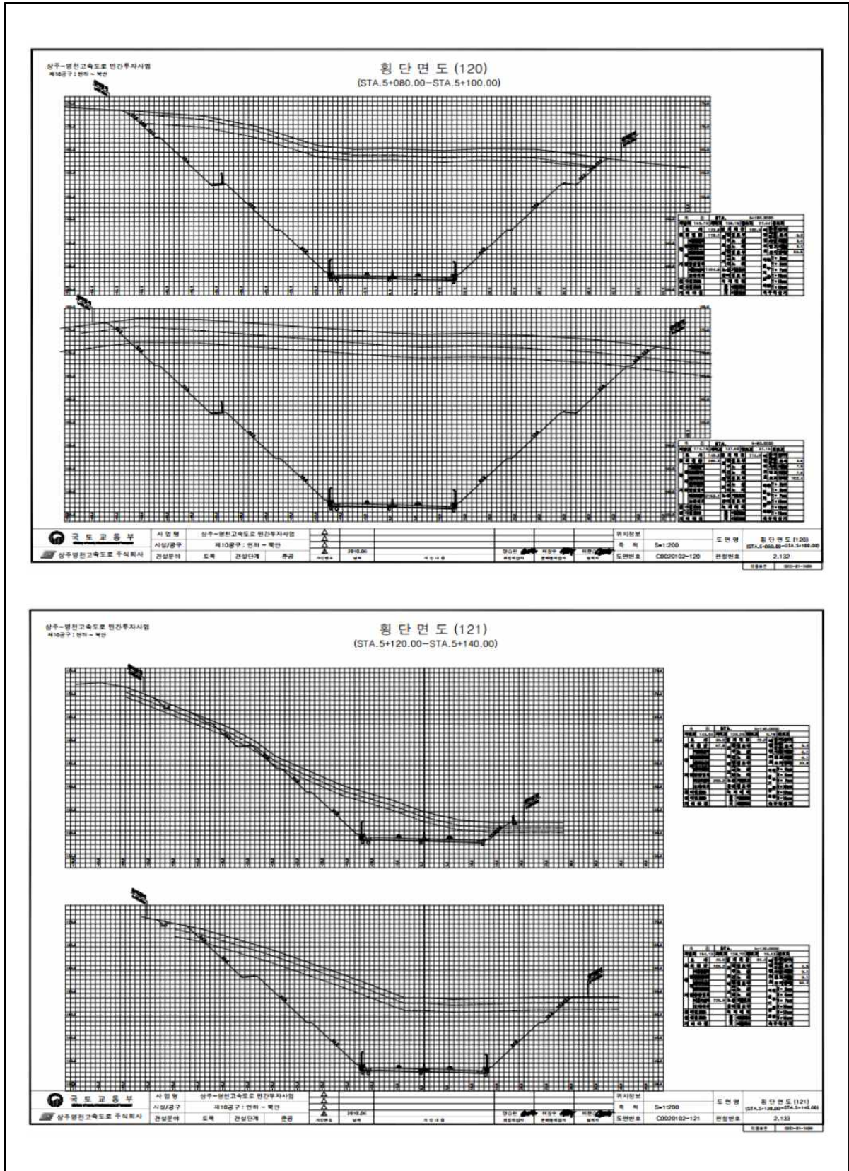
【그림 63.1.5】 표준횡단면도
